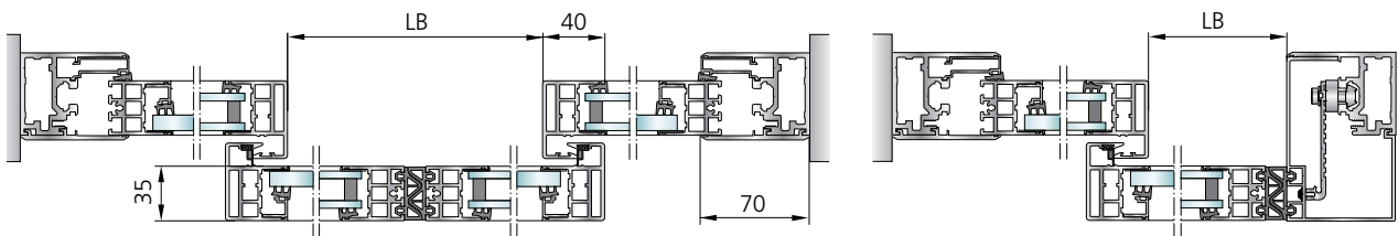
Jamb standard
